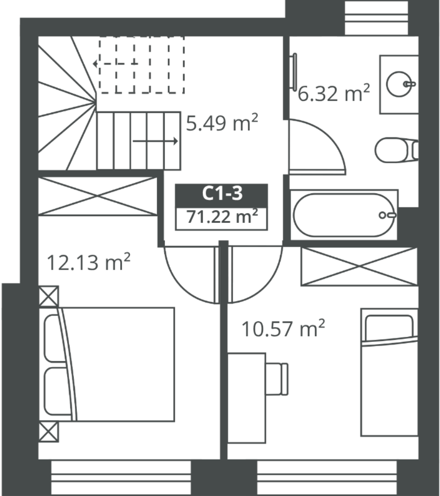
Aukštas 2
