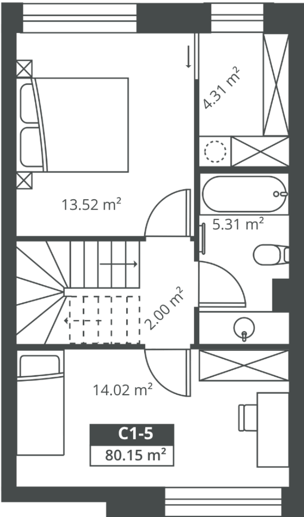
Aukštas 2
